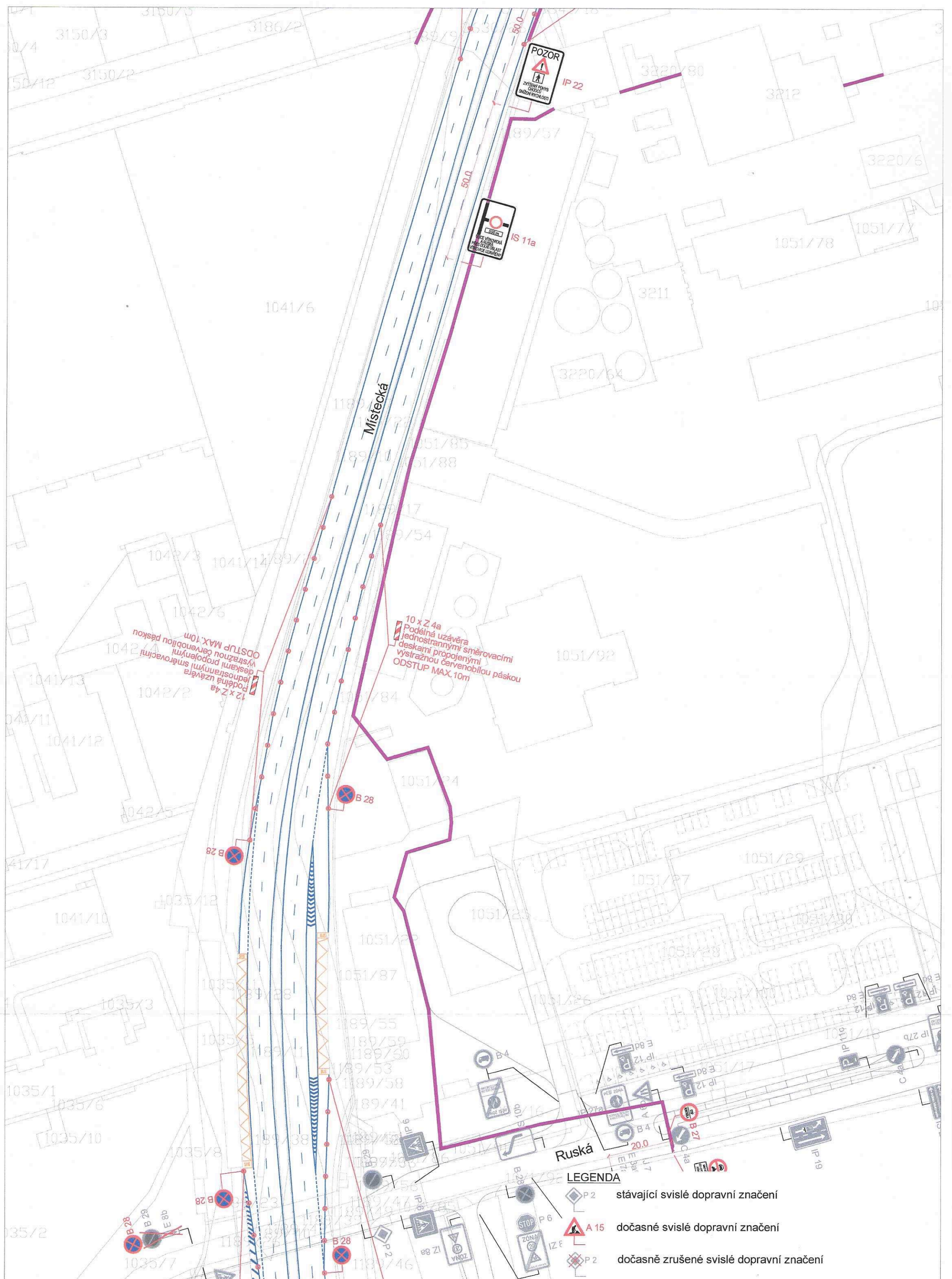
Příloha č.2 situace dopravního značení v místě vjezdu do areálu Dolní oblasti Vítkovice ulice Místecká, ulice Ruská měř. 1:1000
